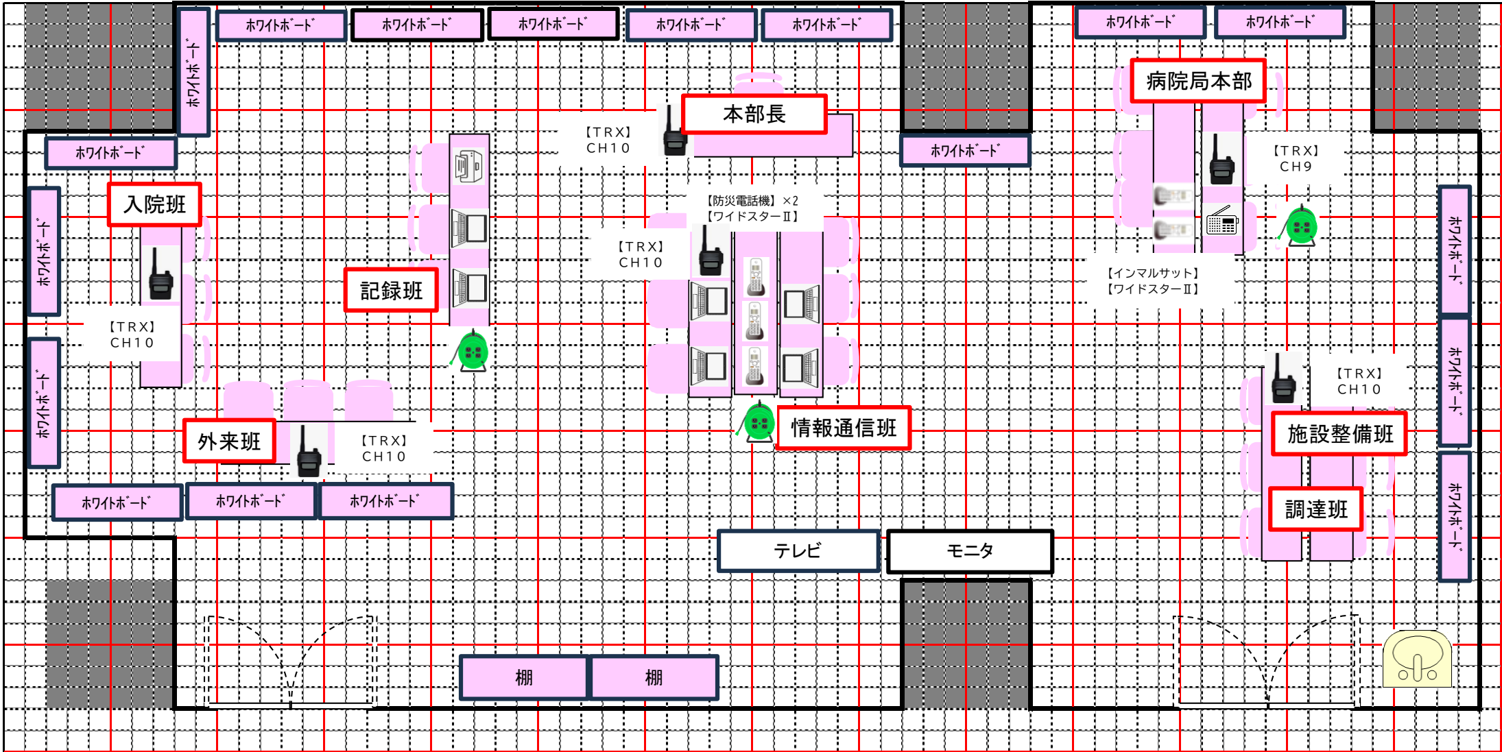
災害対策本部レイアウト図
